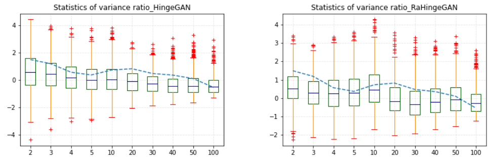
图表71: 标普 500 月频序列: HingeGAN、RaHingeGAN 生成序列方差比率指标
