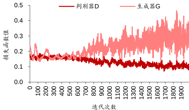
图表49： 标普 500 月频序列：LSGAN 损失函数
